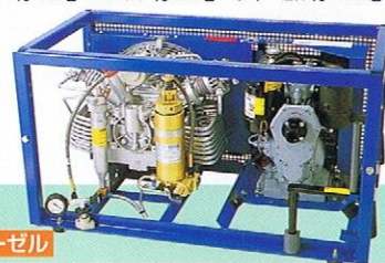
●キャピターノII〈充填〉17分 (12ℓ・200気圧) エアータン容量:201.6ℓ/日 サイズ:L100×W47×H55cm モーター付:89kg エンジン付:91kg ディーゼル付:158kg
